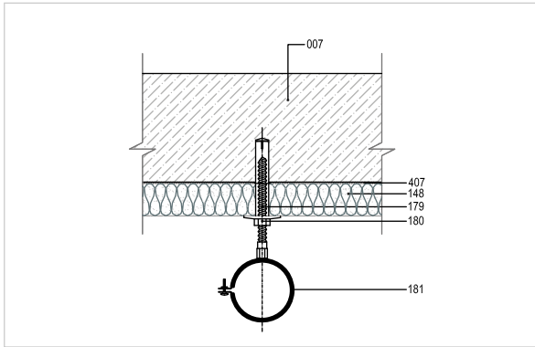
Otopark / Bodrum Kat Tavan Isı Yalıtımı Mekanik Tesisat Taşıma Detayı
